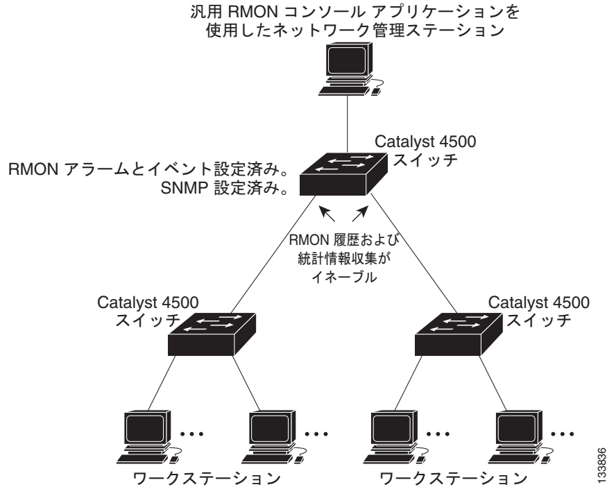
図 68-1 リモート モニタリングの例
