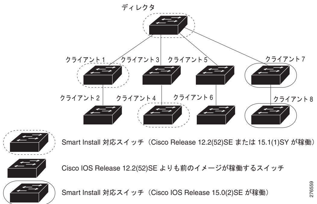
図 1-2 Smart Install クライアントの相互接続
