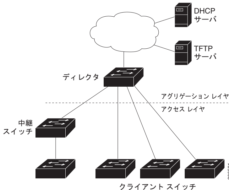
図 1-1 一般的な Smart Install ネットワーク図
