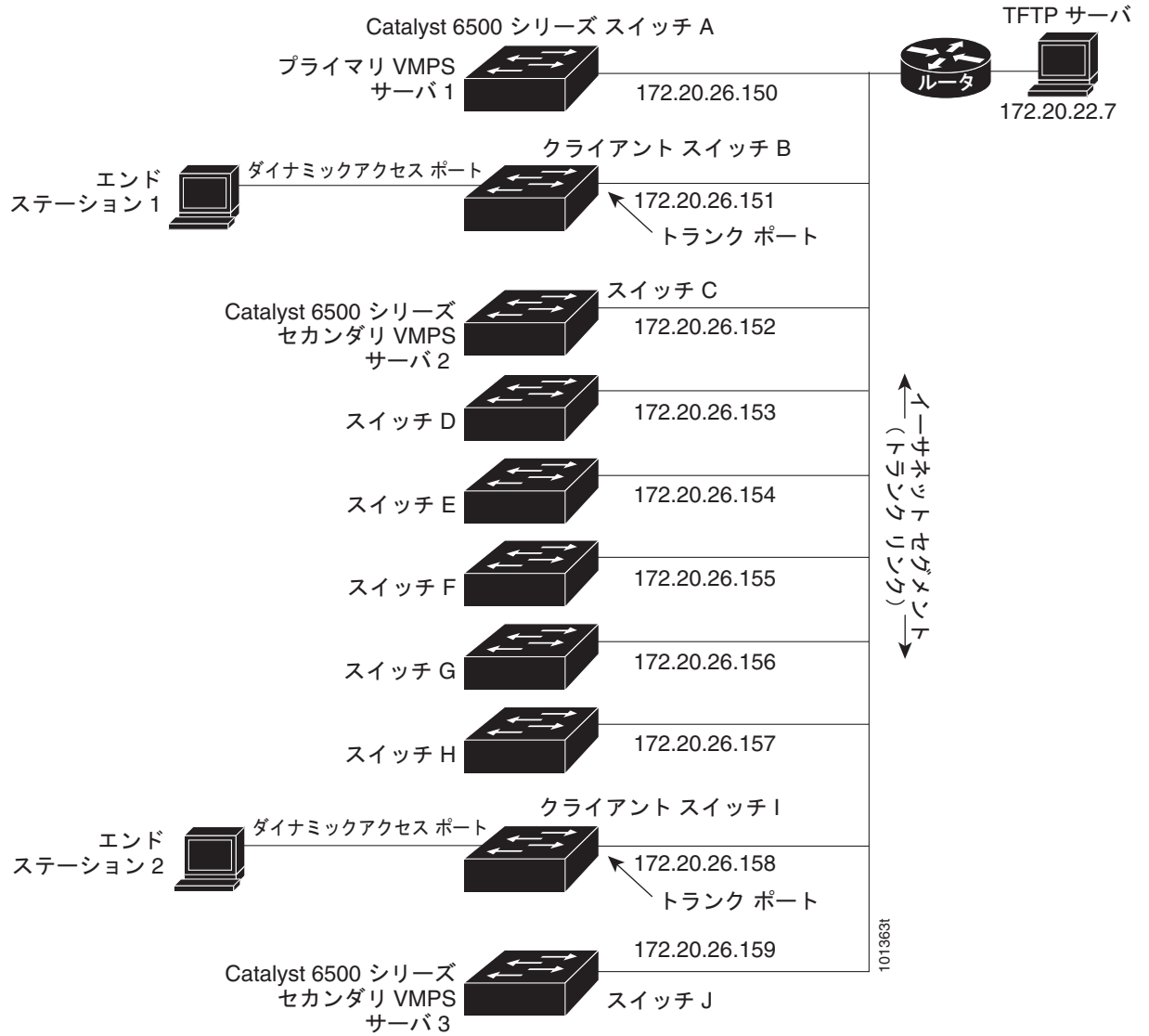
図 14-4 ダイナミック ポート VLAN メンバーシップの構成例
