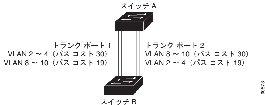
図 14-3 パス コストによってトラフィックが分散される負荷分散トランク
