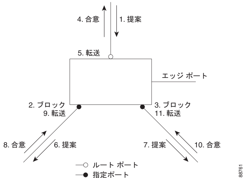
図 18-5 高速コンバージェンス中のイベントのシーケンス
