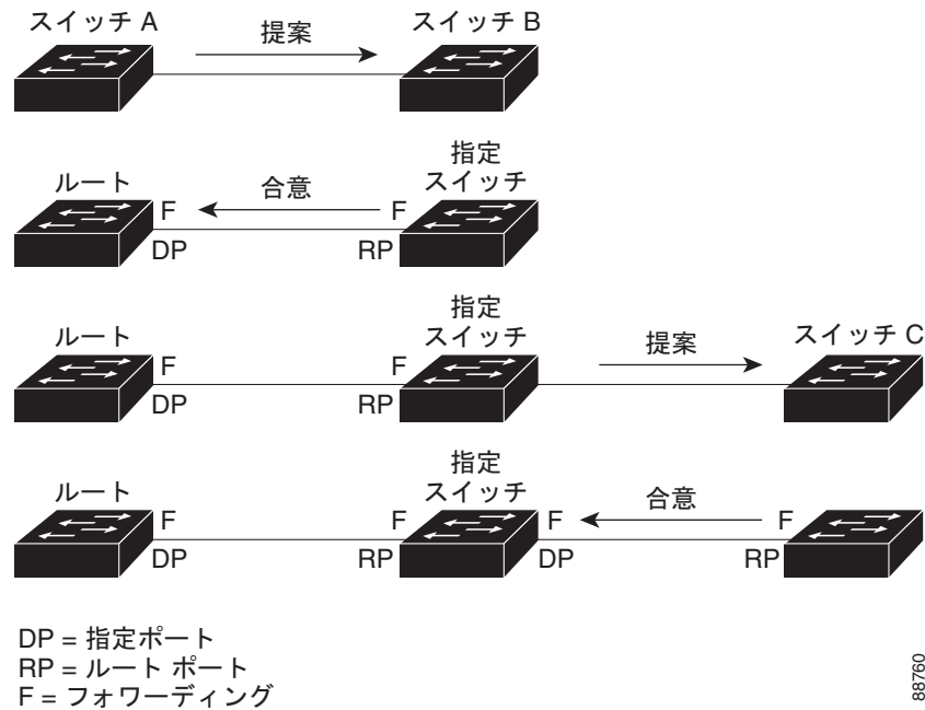
図 18-4 高速コンバージェンスの提案と合意のハンドシェーク
