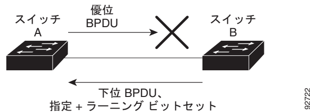
図 18-3 単一方向リンク障害の検出
