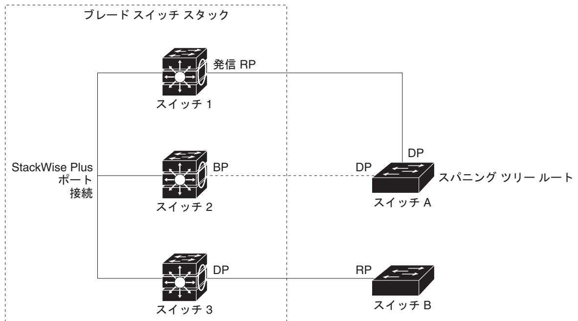
図 18-1 スイッチスタックでのスパニングツリーポートステート
