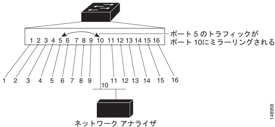
図 30-1 単一スイッチでのローカル SPAN の設定例
