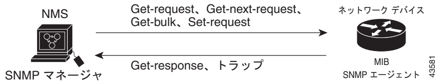
図 33-1 SNMP ネットワーク
