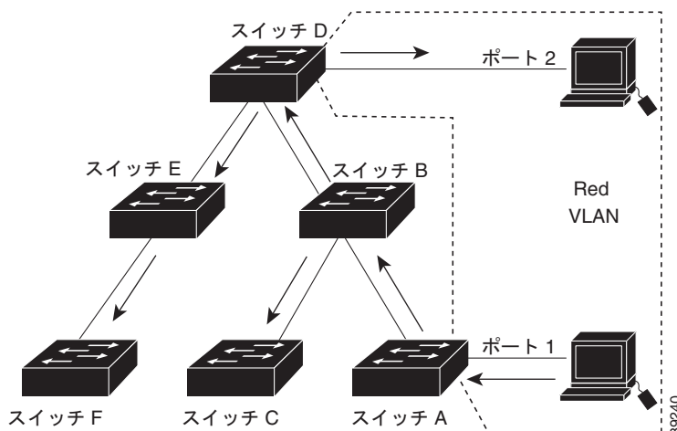
図 13-1 VTP プルーニングを使用しない場合のフラッドイング トラフィック
