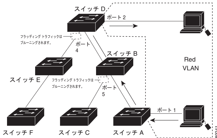
図 13-2 VTP プルーニングによるフラディング トラフィックの最適化
