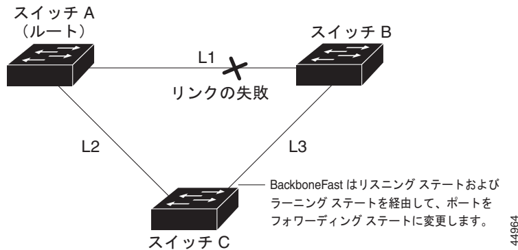
図 19-6 間接リンク障害発生後の BackboneFast の例
