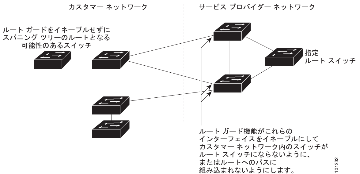
図 19-8 サービスプロバイダー ネットワークのルート ガード
