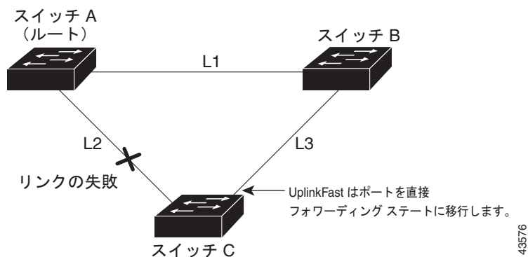
図 19-4 直接リンク障害発生後の UplinkFast の例
