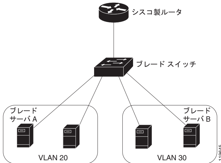
図 10-1 レイヤ 2 スイッチによる VLAN の接続
