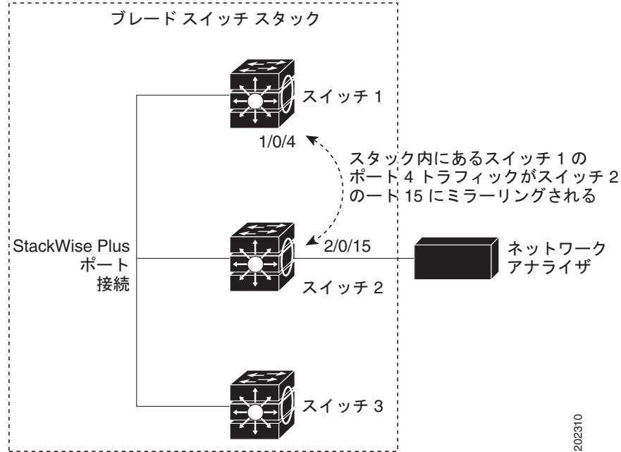
図 30-2 単一スイッチ スタックでのローカル SPAN の設定例
