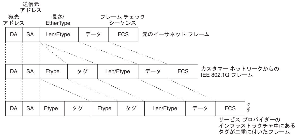
図 16-2 元の（標準）、IEEE 802.1Q、および二重タグ付きイーサネット パケットの形式
