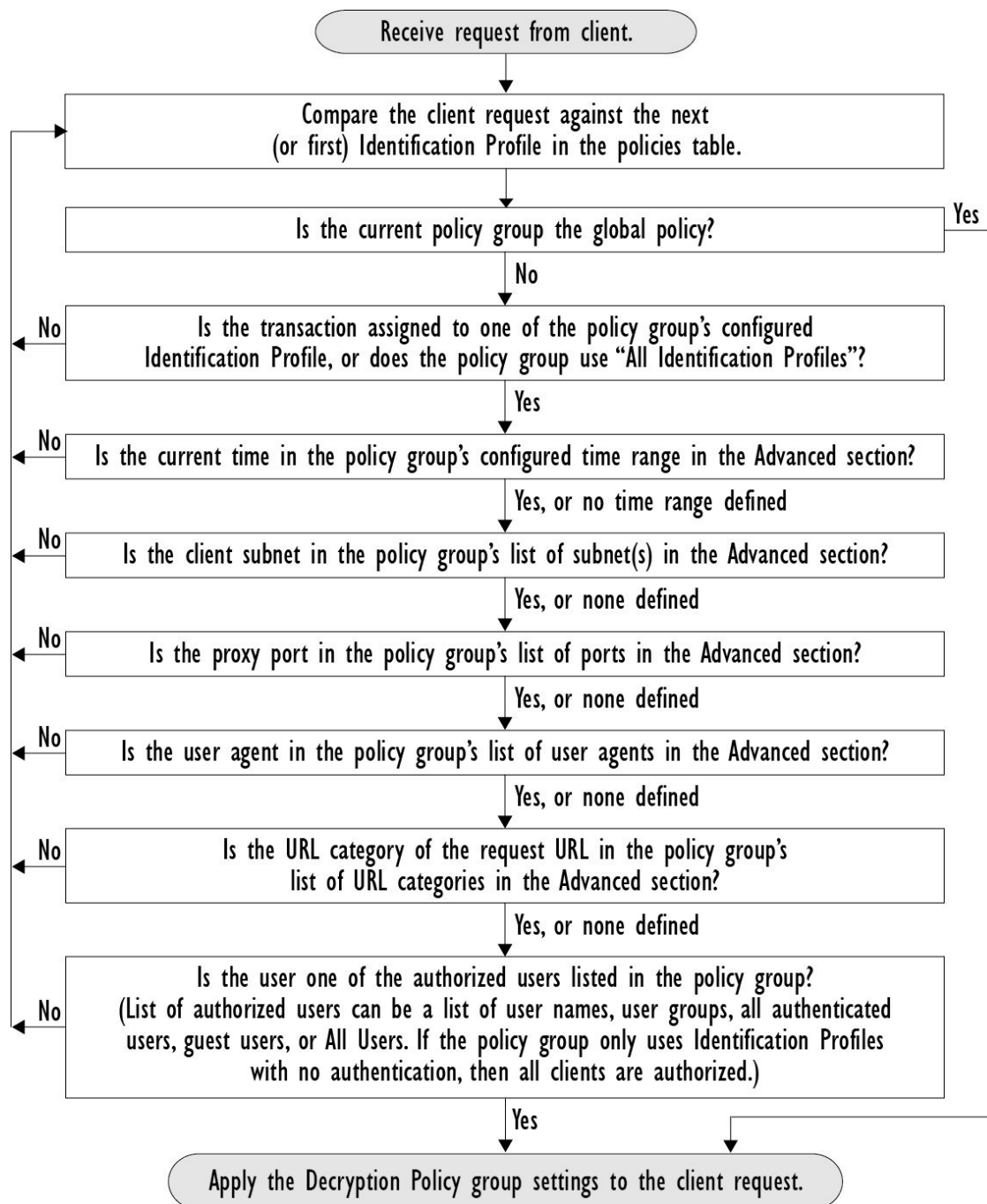
Figure 5: 復号ポリシーのポリシー グループ トランザクション フロー
