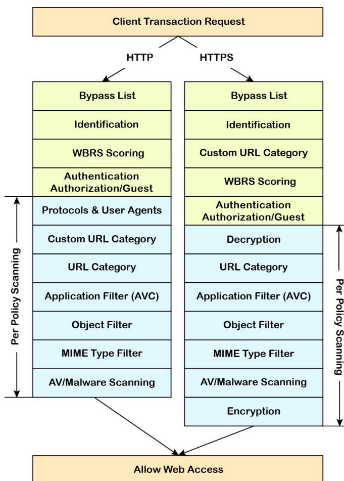
Figure 7: HTTP/HTTPS トランザクション フロー
