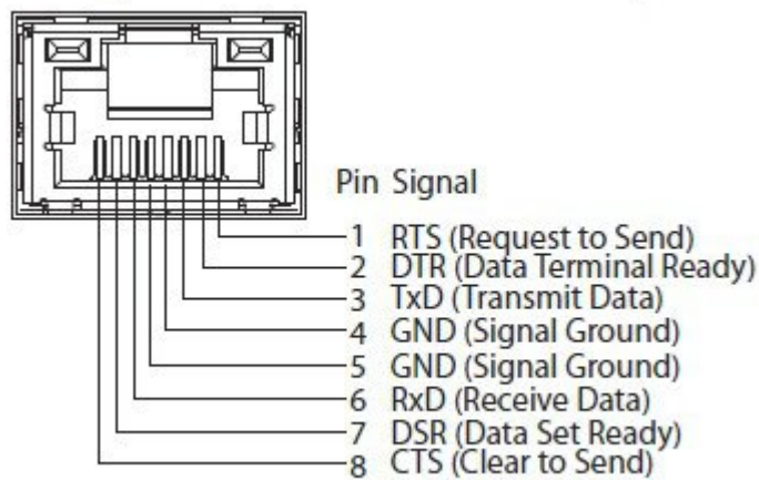
Figure 1: 80 および 90 シリーズ ハードウェアでのシリアルポートのピン割り当ての詳細
