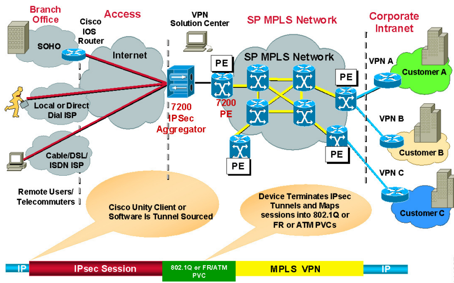
図 8: VRF 対応 IPsec 2 ボックス ソリューション
