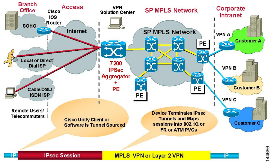
図 7: VRF 対応 IPsec 1 ボックス ソリューション
