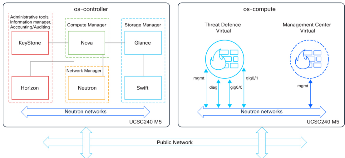
図 2: OpenStack で Firewall Management Center Virtual を使用したトポロジの例
