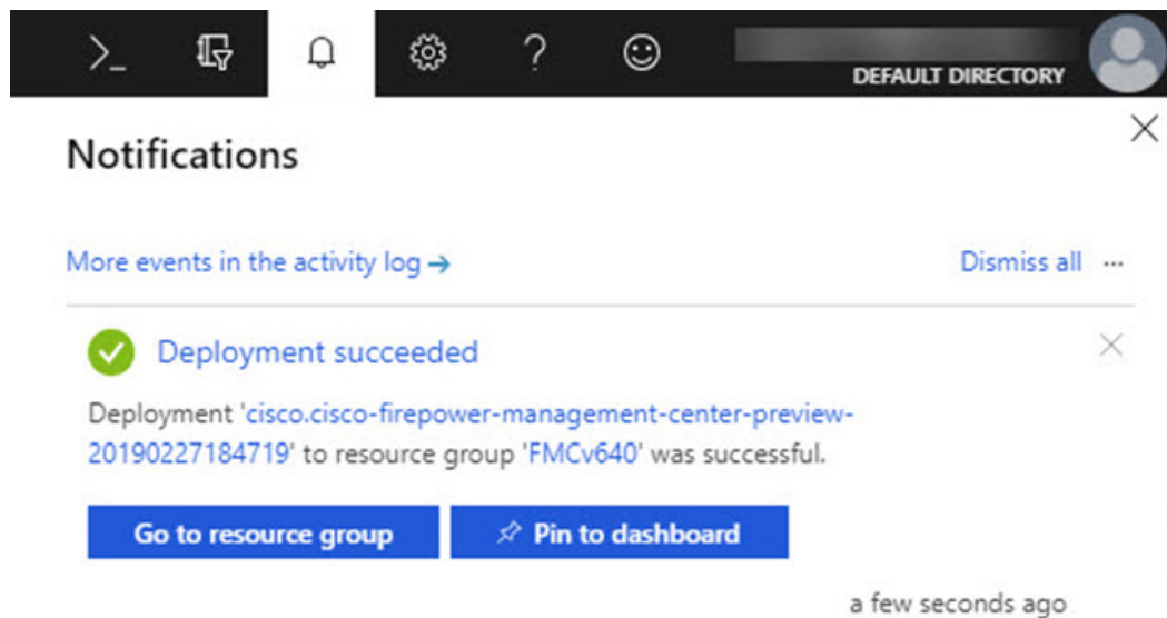
図 1: Azure 通知
