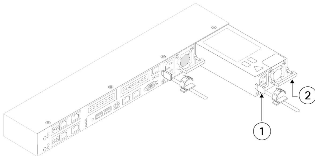
図 36: AC 電源装置の取り外しと交換
