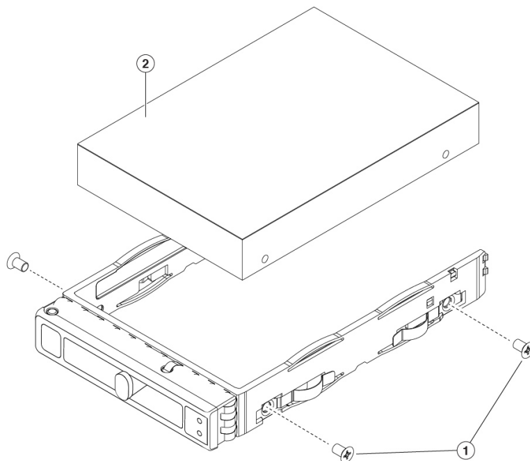
図 35: ドライブトレイの取り外し
