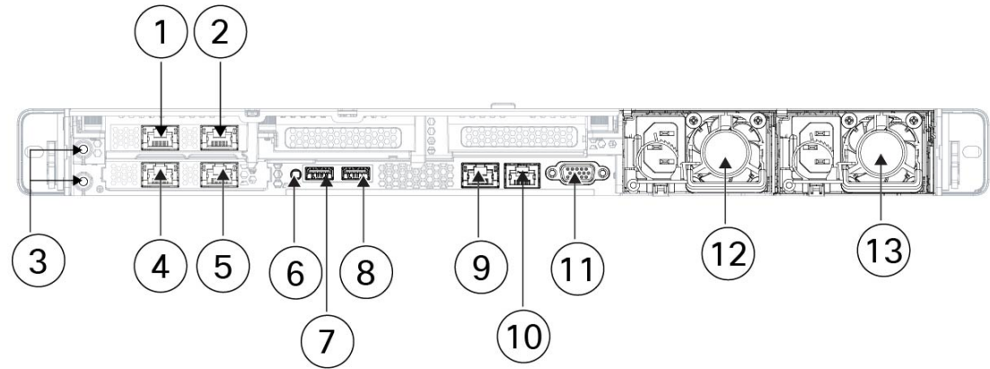
図 9: 1700、2700、および 4700 の背面パネル
