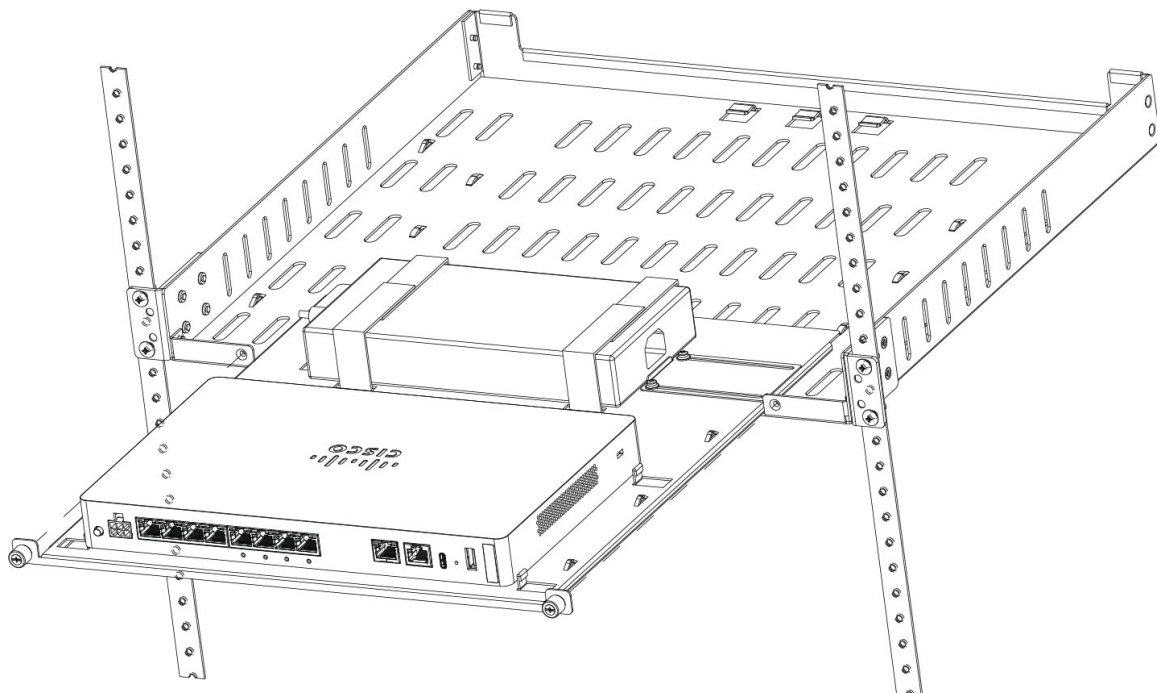
図 8: ラックマウントシェルフへのスライド式ラックトレイの取り付け
