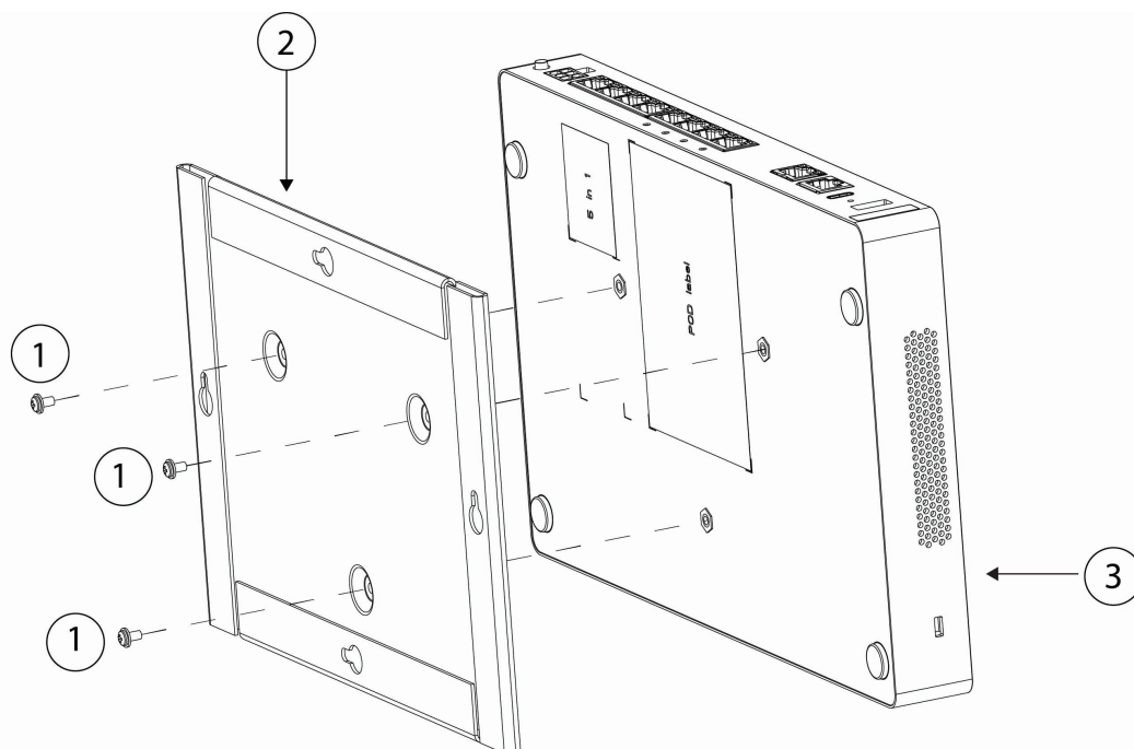
図 3: シャーシへの壁面取り付けブラケットの取り付け
