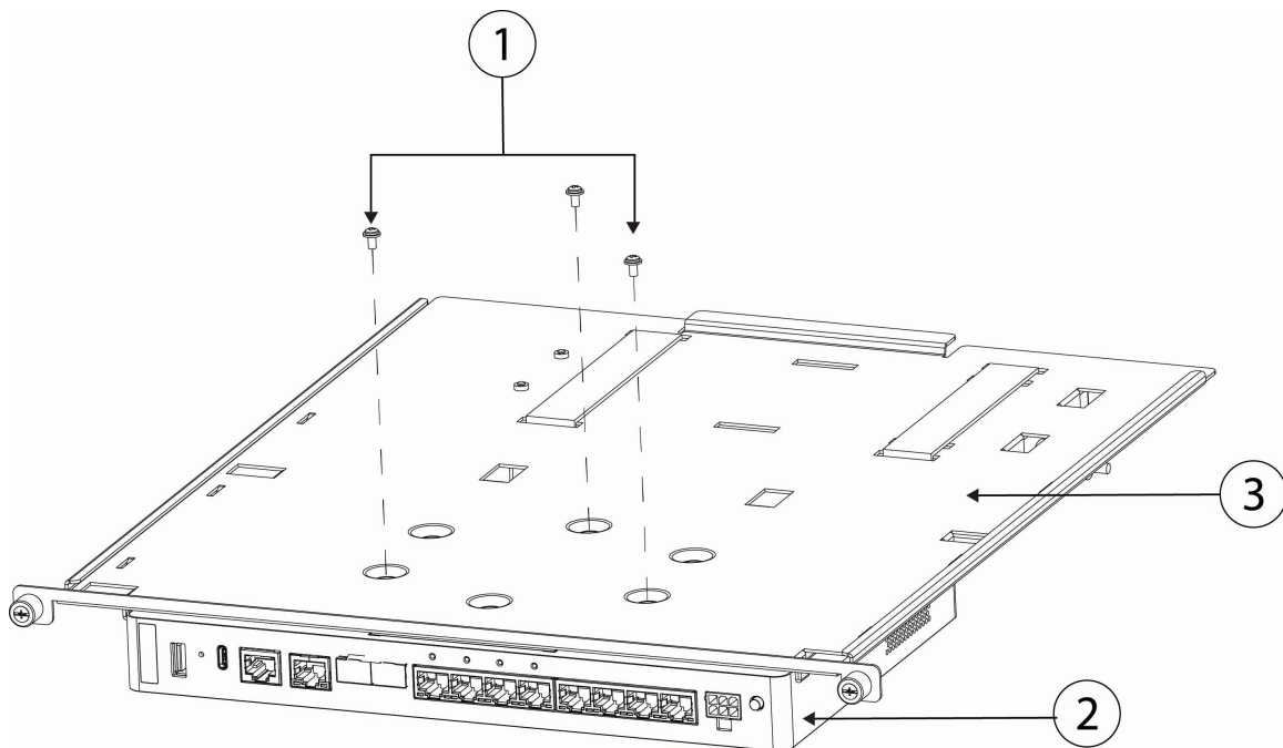
図 6: シャーシへのスライド式ラックトレイの取り付け
