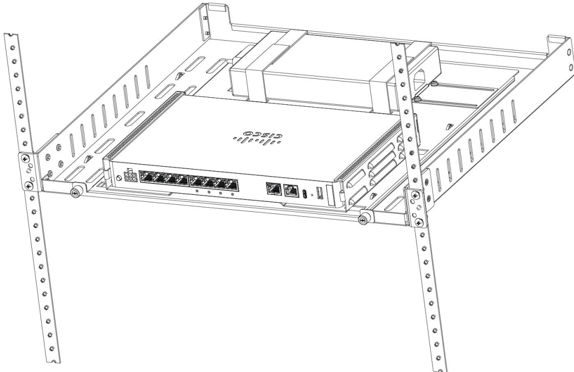
図 9: ラックマウントシェルフに取り付けられたスライド式ラックトレイ
