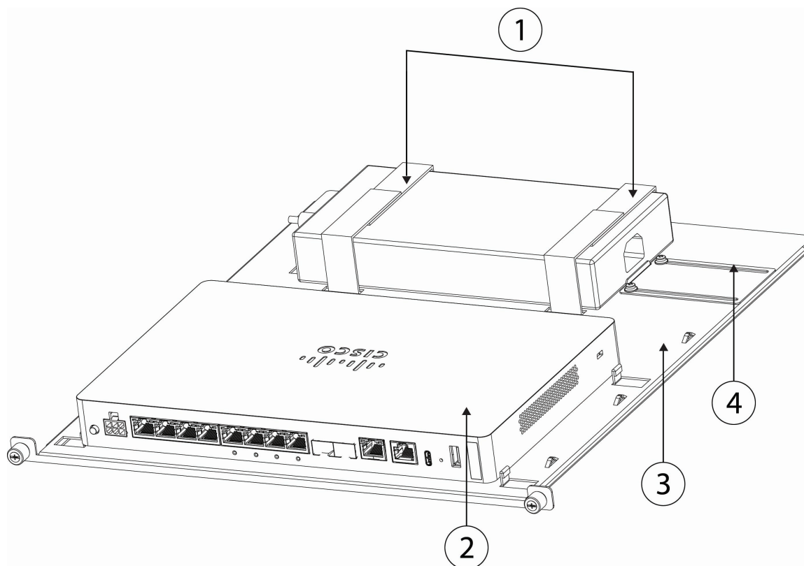
図 7: スライド式ラックトレイへの電源の取り付けとベルクロストラップの締め付け
