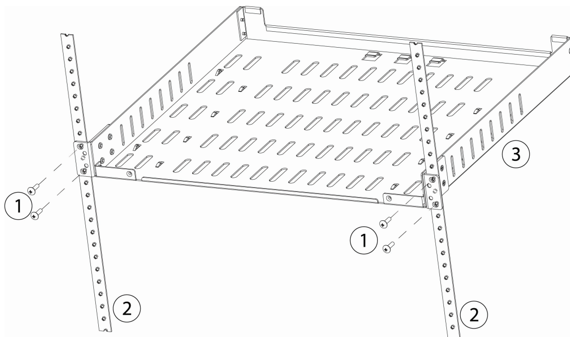
図 5: ラックへのラックマウントシェルフの取り付け
