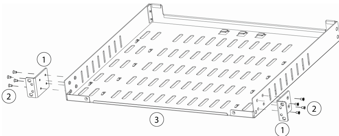
図 4: ラックマウントシェルフへのラックマウントブラケットの取り付け
