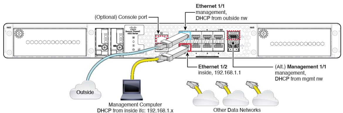
図 2: Cisco Secure Firewall 4200 のケーブル接続
