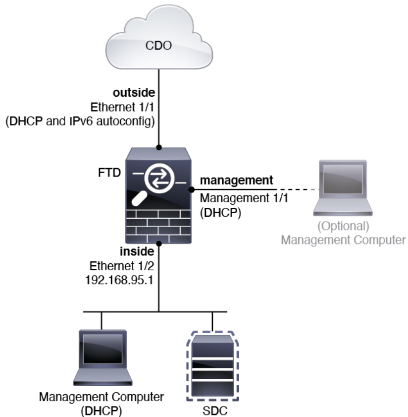
図 6: 推奨されるネットワーク展開（オンプレミスの SDC）
