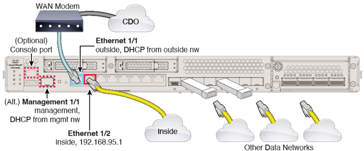
図 2 : Cisco Secure Firewall 3100 のケーブル接続
