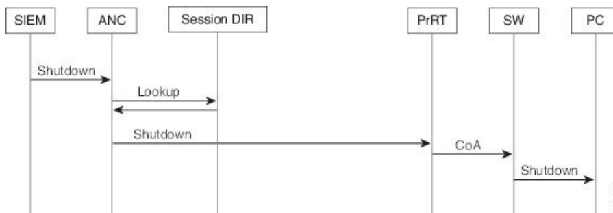
図 1: ANCのシャットダウンフロー
