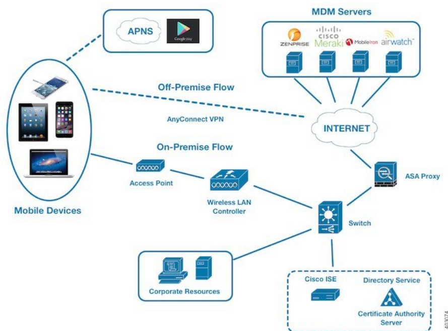
図 34: MDM の Cisco ISE との相互運用性
