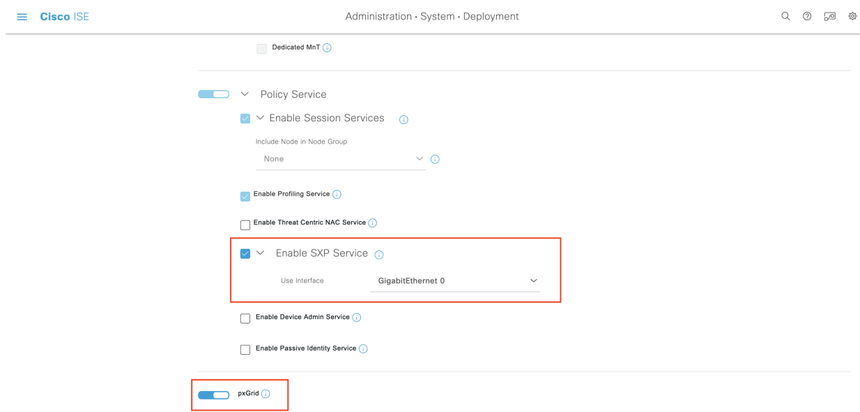
図 71: SXP および pxGrid サービスの有効化
