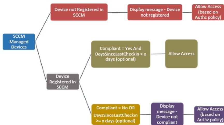
図 39: SCCM のワークフロー
