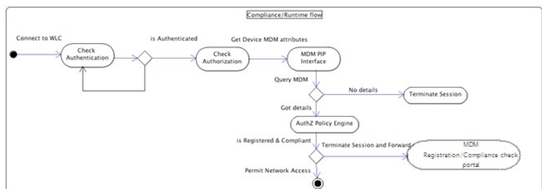
図 35: Cisco ISE での MDM プロセスフロー
