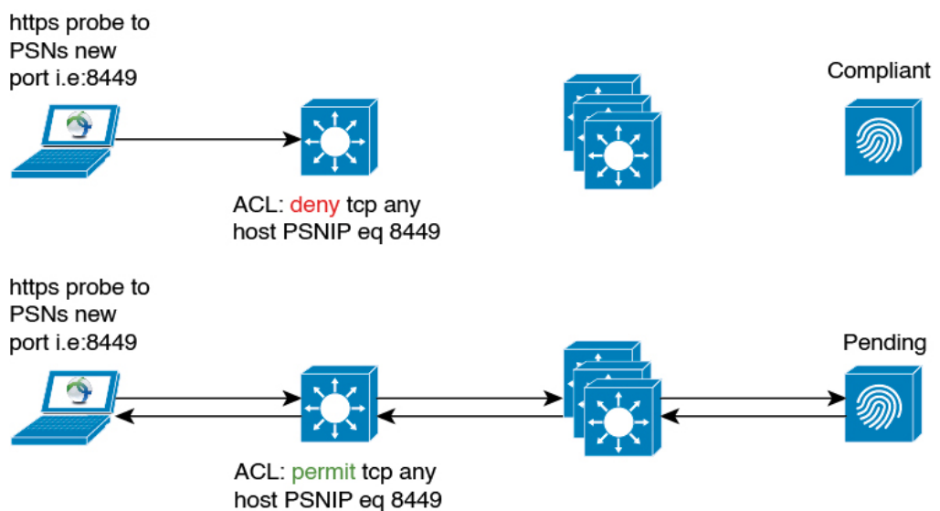
図 80: ポスチャ状態の同期
