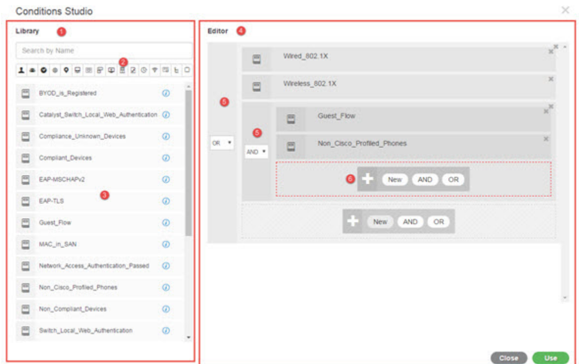
図 58: [条件スタジオ (Conditions Studio) ]
