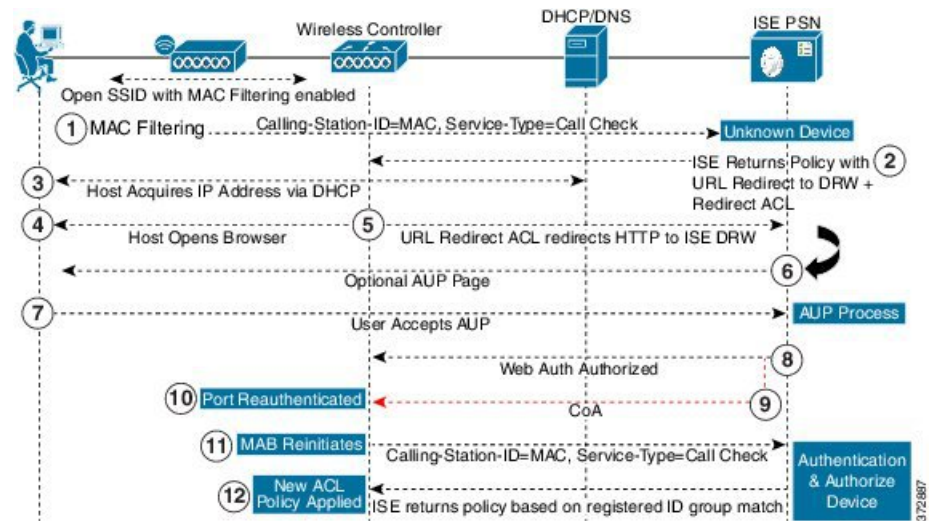
図 14: ワイヤレス デバイス登録 Web 認証フロー
