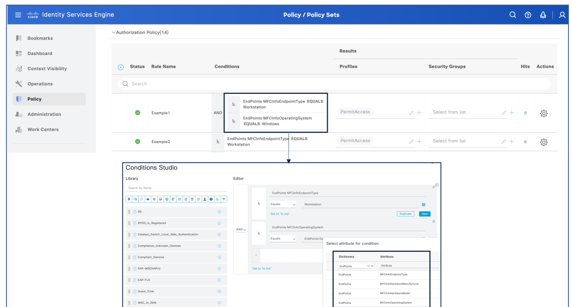
図 27: 多要素分類属性を使用する条件付きの認証ポリシー
