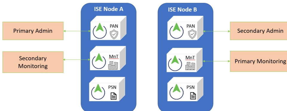
図 1: Cisco ISE 2 ノード管理展開
