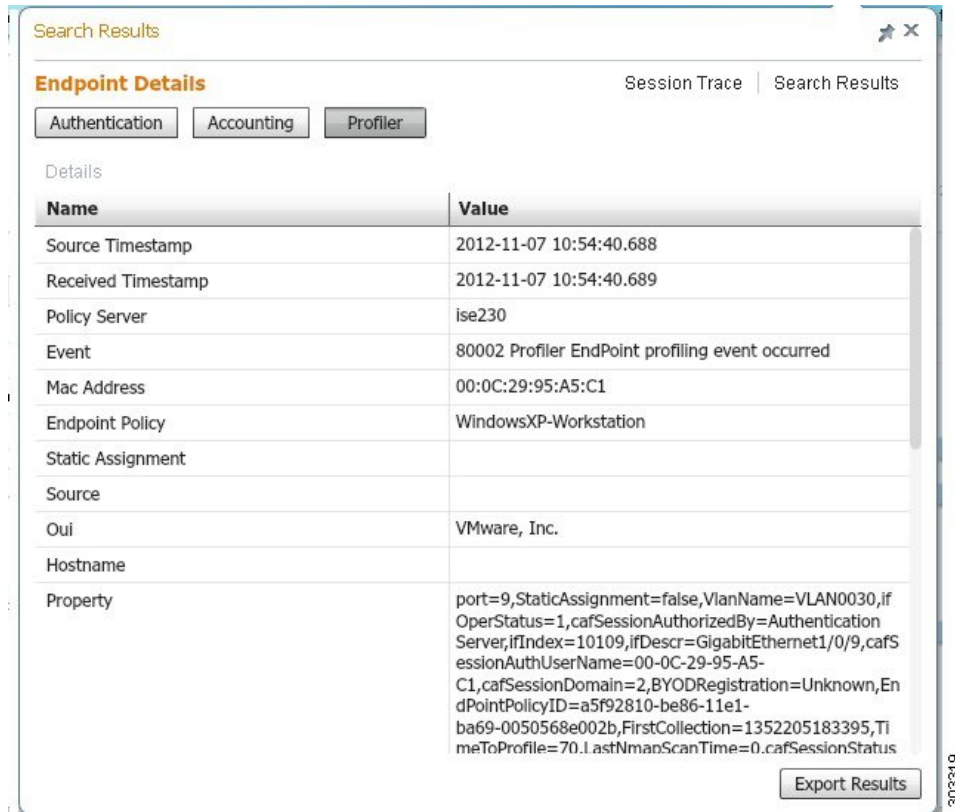
図 14: エンドポイントの詳細
