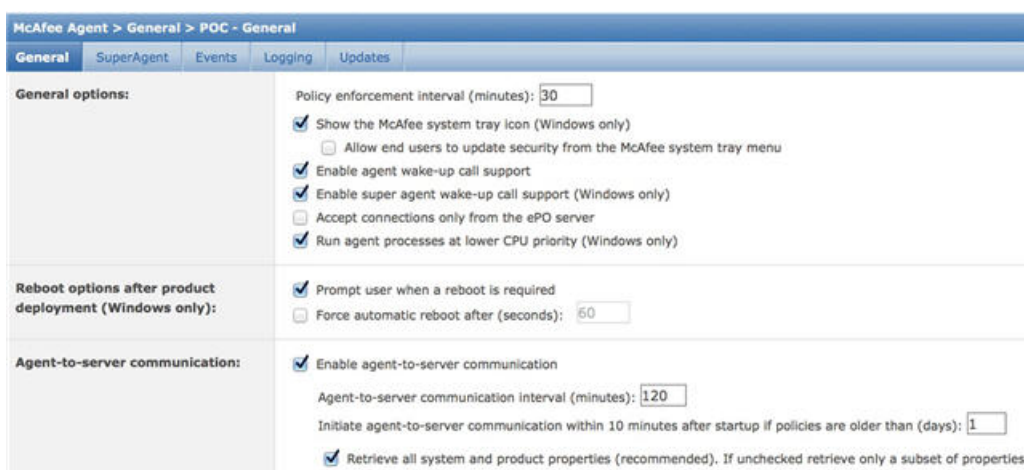
図 12: McAfee ePO Agent の推奨されるオプション
