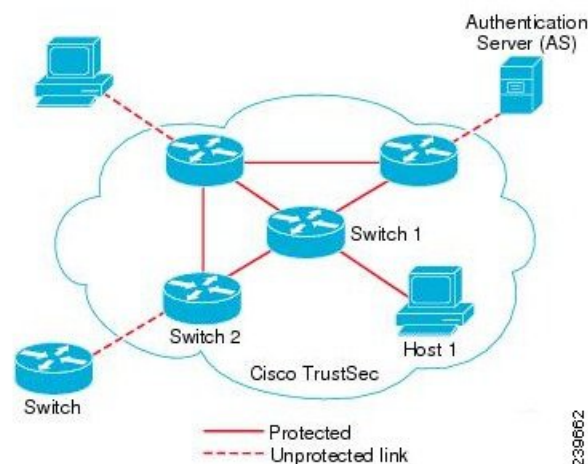
図 52: TrustSec アーキテクチャ
