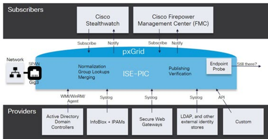
図 24: パッシブ ID サービス フロー
