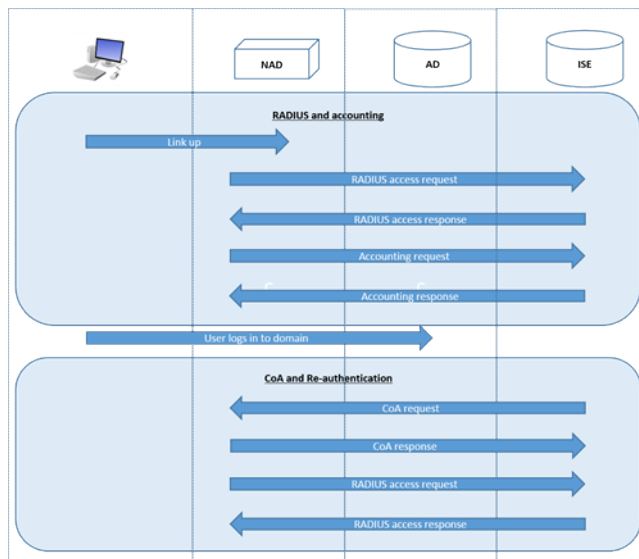
図 18: Easy Connect 適用モードの詳細フロー
