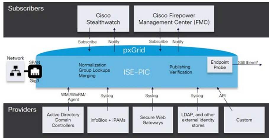
図 20: 全体的なフロー
