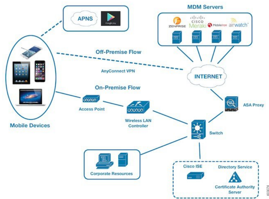
図 30: MDM の Cisco ISE との相互運用性
