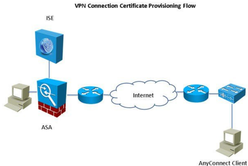
図 10: ASA VPN ユーザーの証明書プロビジョニング
