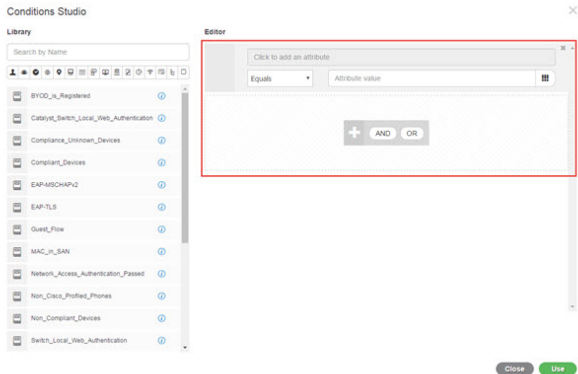
図 42: 条件スタジオ：新しい条件の作成
