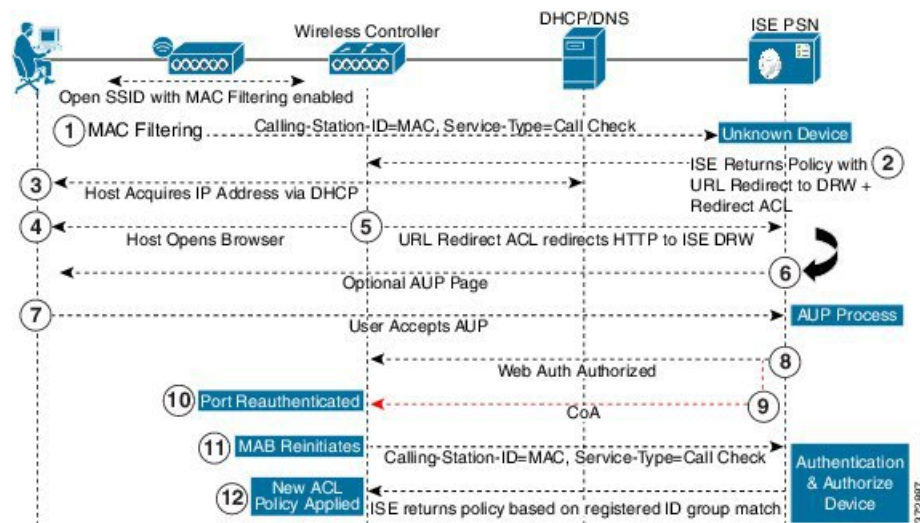
図 13: ワイヤレス デバイス登録 Web 認証フロー
