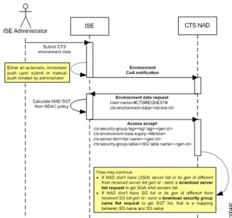
図 47: 環境 CoA 通知のフロー
