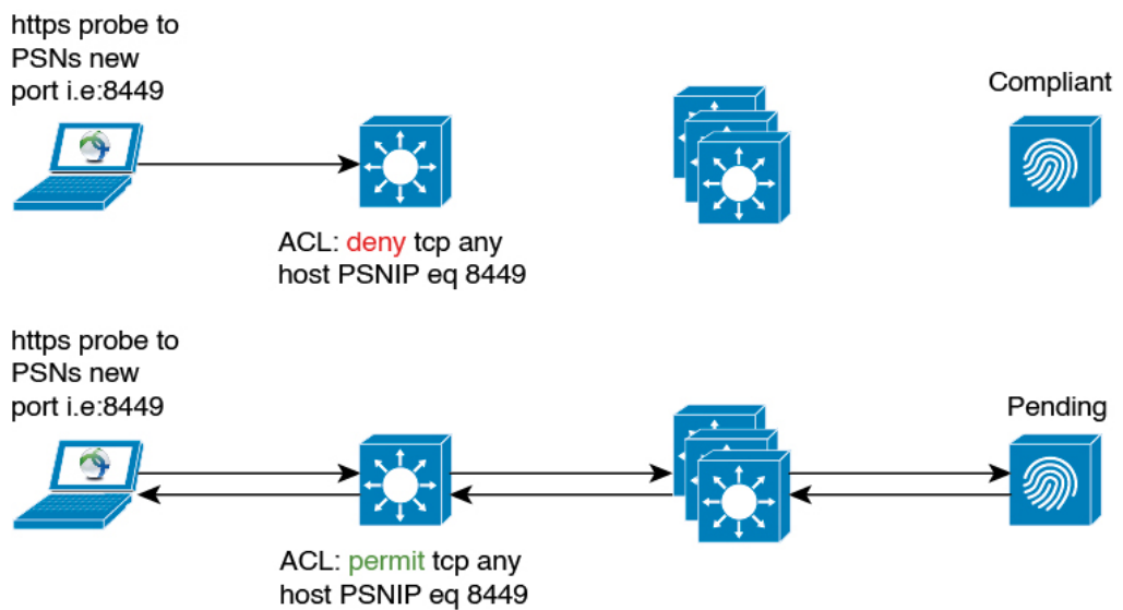
図 62: 双方向ポスタチャフロー
