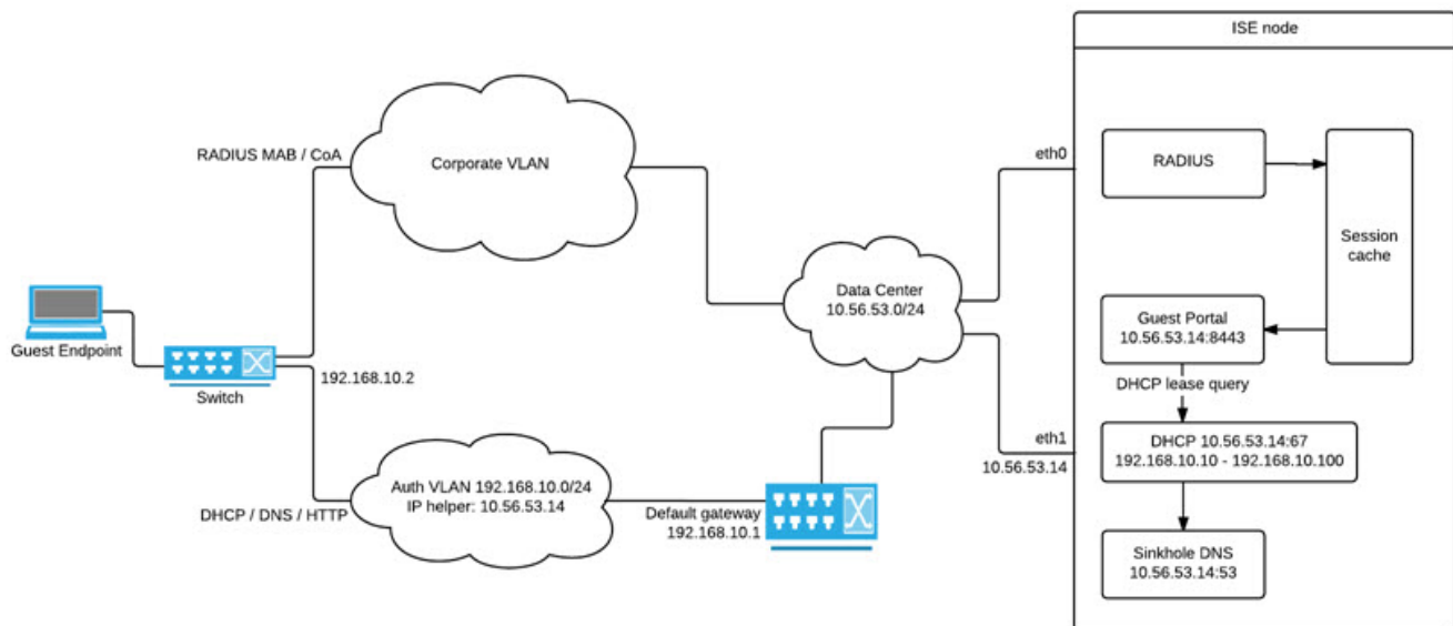
図 31: IP ヘルパーを備えた認証 VLAN 構成
