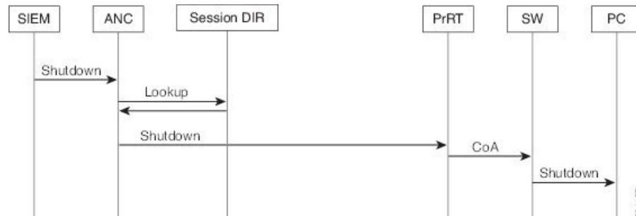
図 11: ANC のシャットダウンフロー
