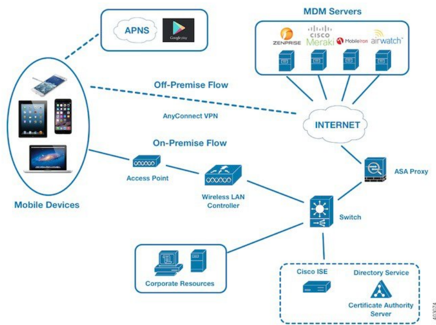
図 32: MDM の Cisco ISE との相互運用性
