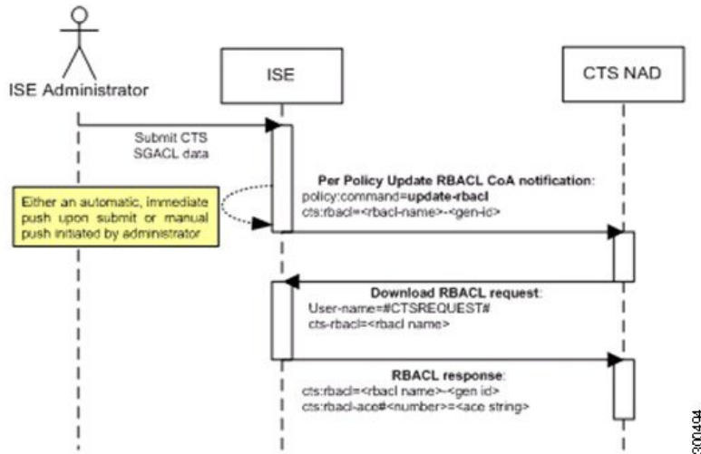
図 48: SGACL コンテンツ更新のフロー
