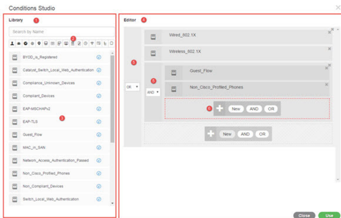
図 40: 条件スタジオ
