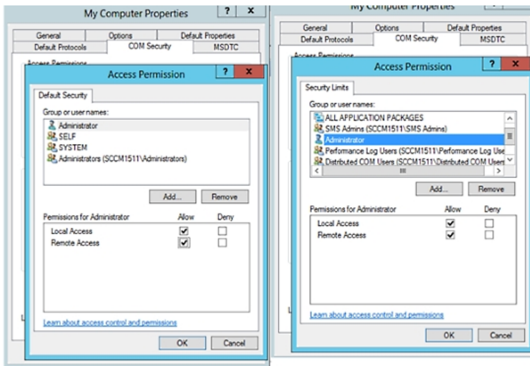
図 15: [アクセス権限 (Access Permissions)] に対するローカルアクセスとリモートアクセス
