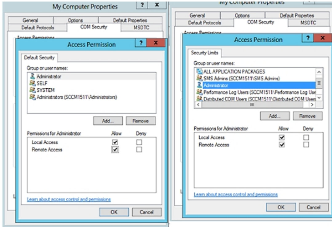
図 36: [アクセス権限 (Access Permissions)] に対するローカルアクセスとリモートアクセス
