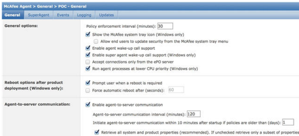
図 27: McAfee ePO Agent の推奨されるオプション
