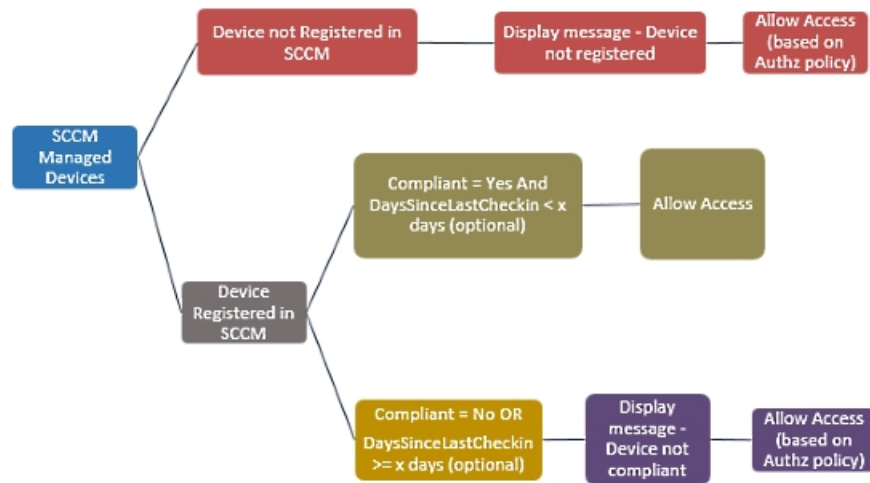
図 35: SCCM のワークフロー
