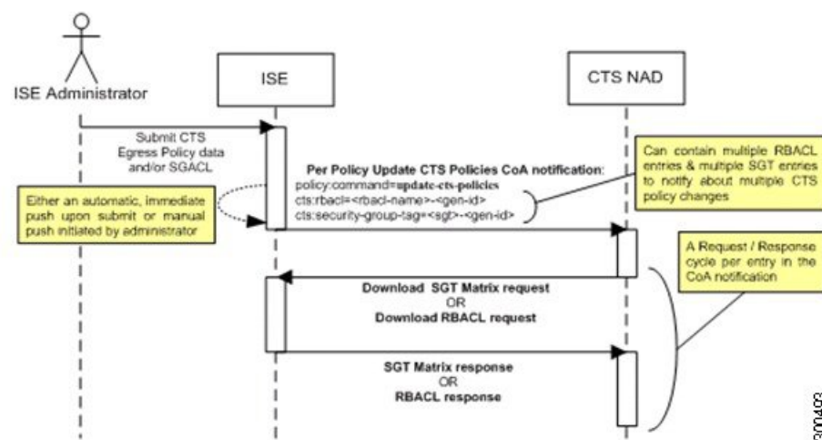
図 49: ポリシーの CoA 通知のフロー
