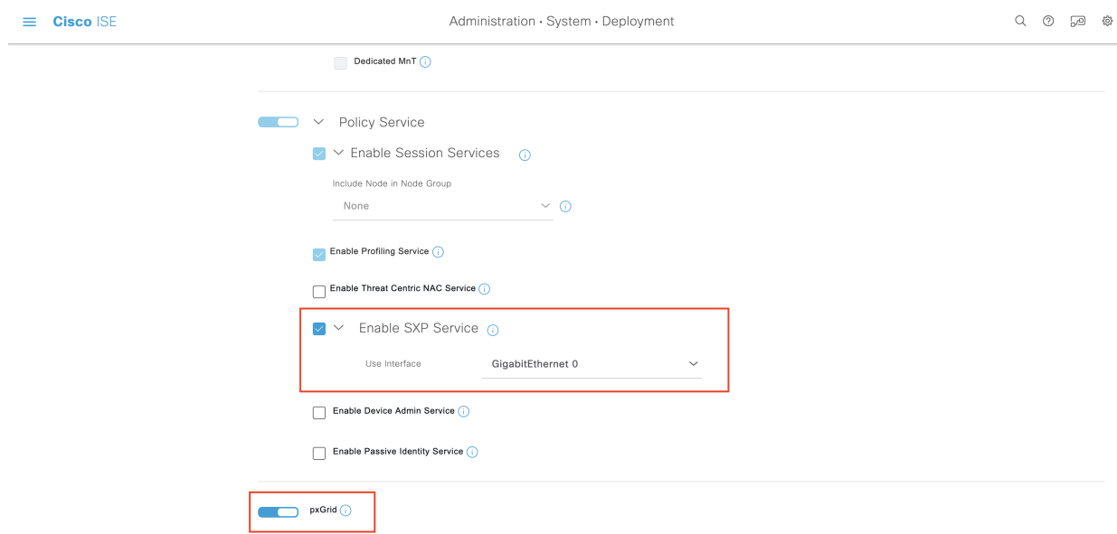
図 53: SXP および pxGrid サービスの有効化
