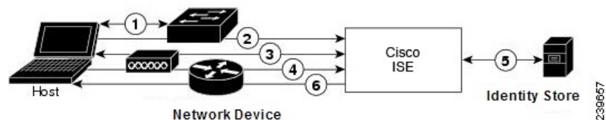
図 43: EAP を使用しない RADIUS ベースの認証
