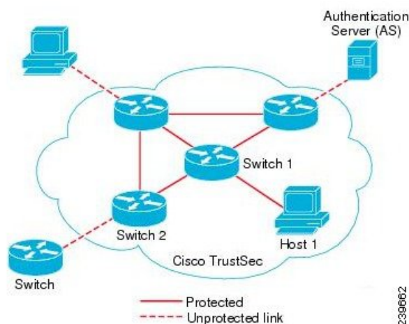
図 45: TrustSec アーキテクチャ
