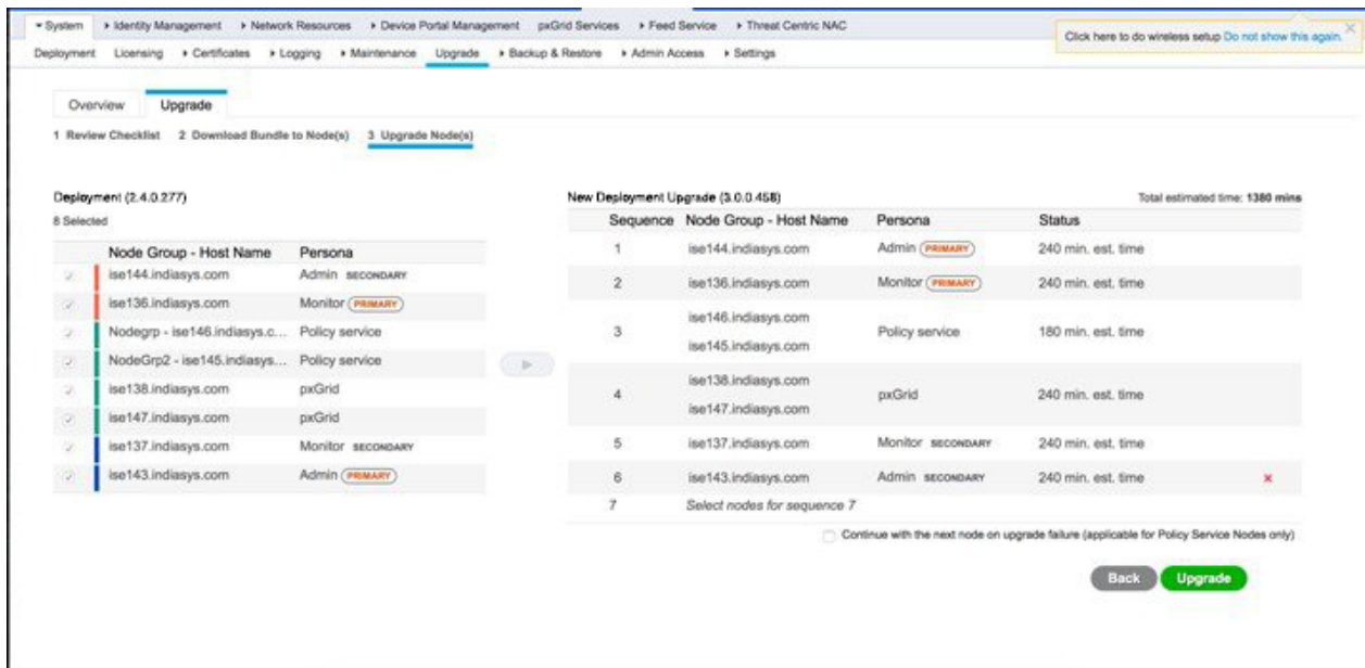
図 1: 各ノードの選択したりポジトリを表示するアップグレードウィンドウ
