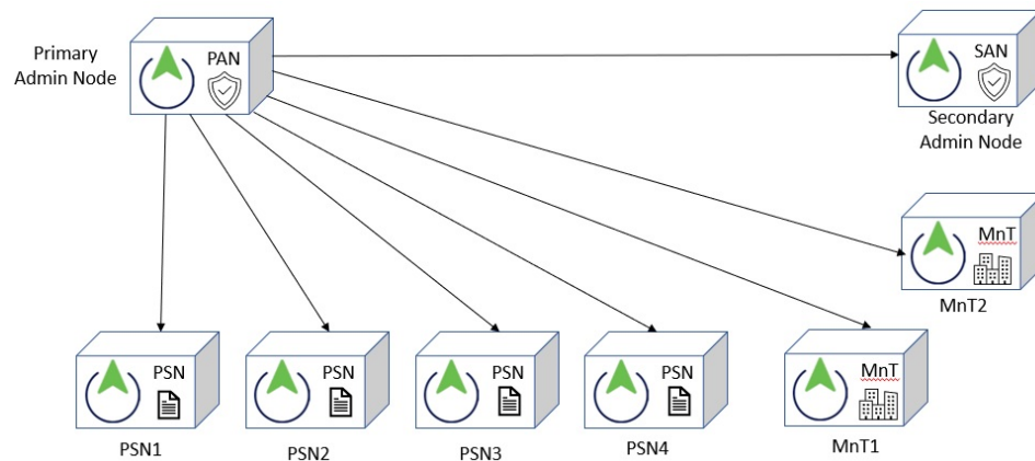
図 4: アップグレード前の Cisco ISE 展開
