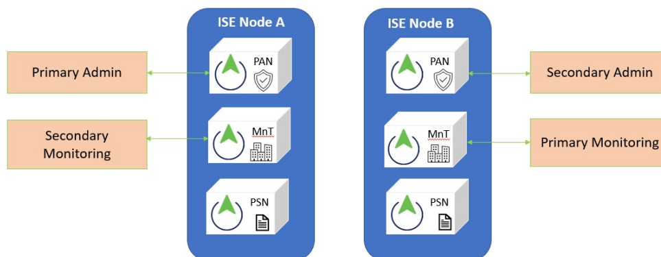
図 3: Cisco ISE 2 ノード管理展開
