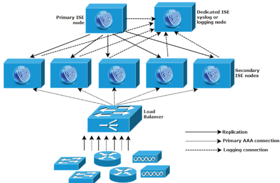
図 4: ロードバランサを使用した Cisco ISE での大規模なネットワークデプロイメント
