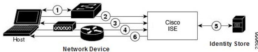
図 8: EAP を使用する RADIUS ベースの認証
