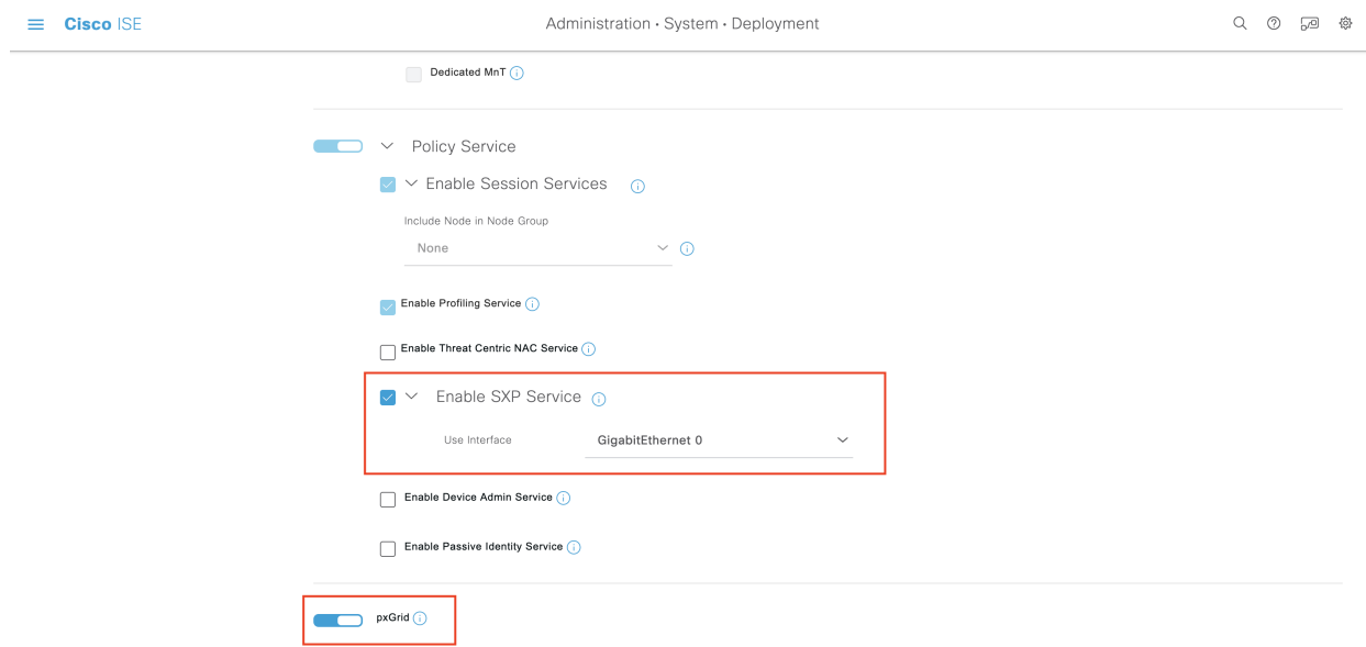
図 17: SXP および pxGrid サービスの有効化
