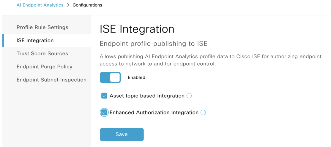
図 3: Cisco AI エンドポイント分析の ISE 統合設定
