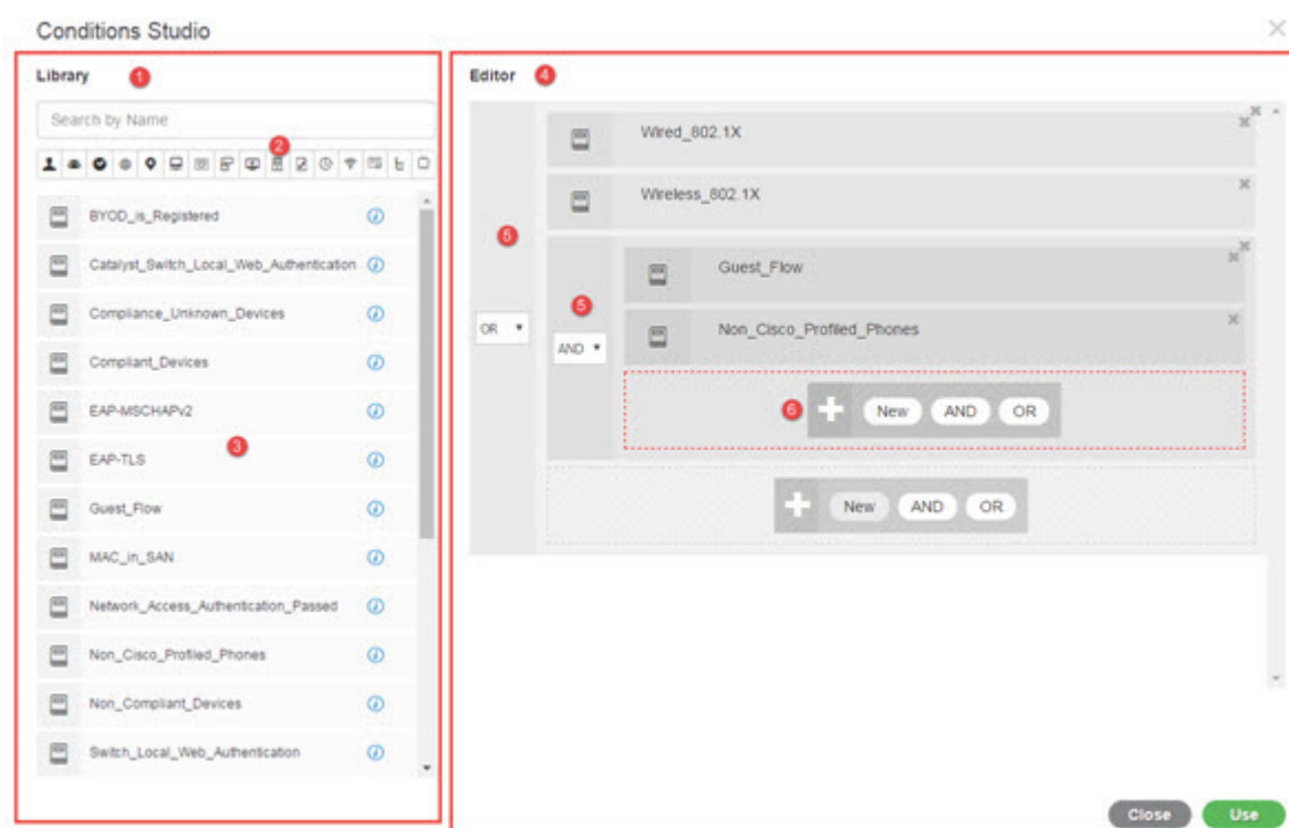
図 4:[条件スタジオ (Conditions Studio) ]
