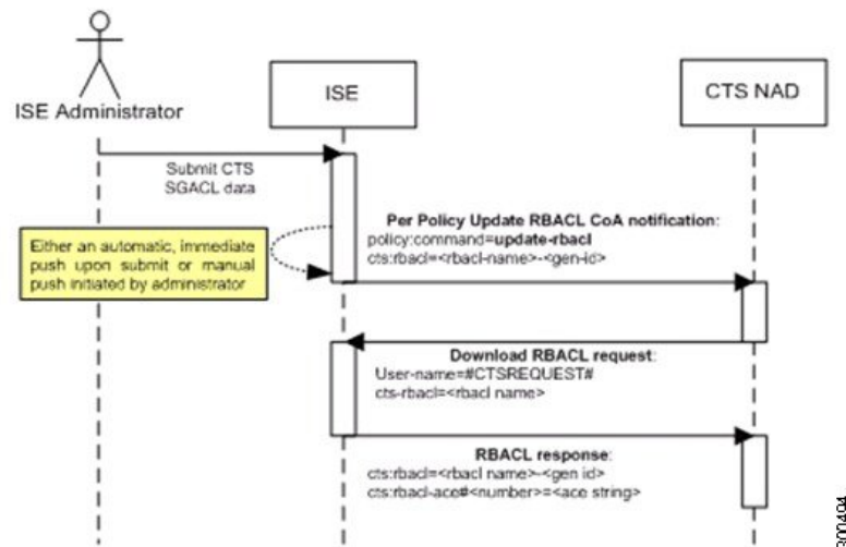
図 12: SGACL コンテンツ更新のフロー
