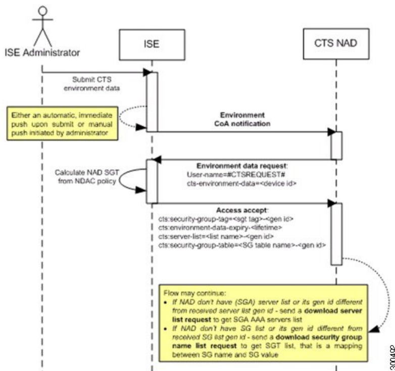
図 11: 環境 CoA 通知のフロー
