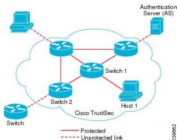
図 9: TrustSec アーキテクチャ
