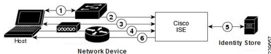
図 7: EAP を使用しない RADIUS ベースの認証
