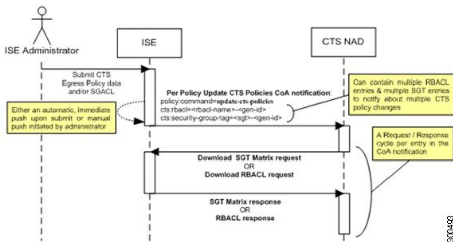
図 13: ポリシーの CoA 通知のフロー
