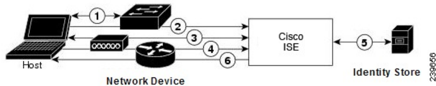
Figure 57: EAP を使用する RADIUS ベースの認証
