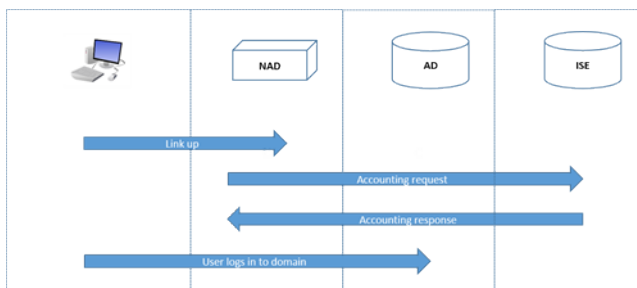
図 28: Easy Connect 可視性モードのフロー
