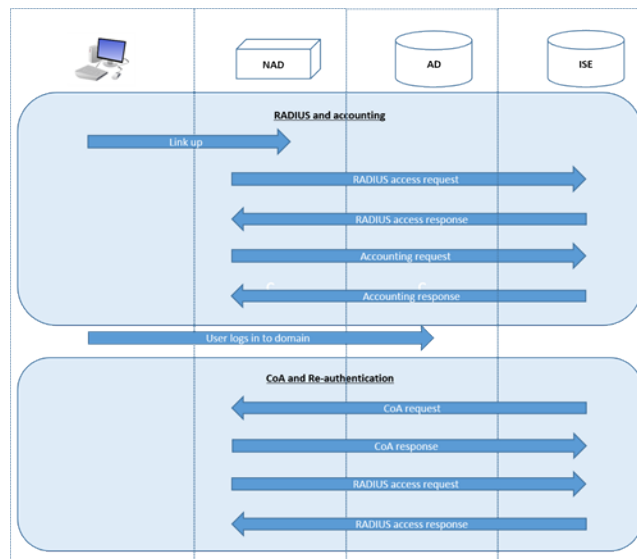
図 27: Easy Connect 適用モードの詳細フロー
