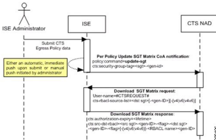
図 63: SGT マトリクスの更新 CoA のフロー
