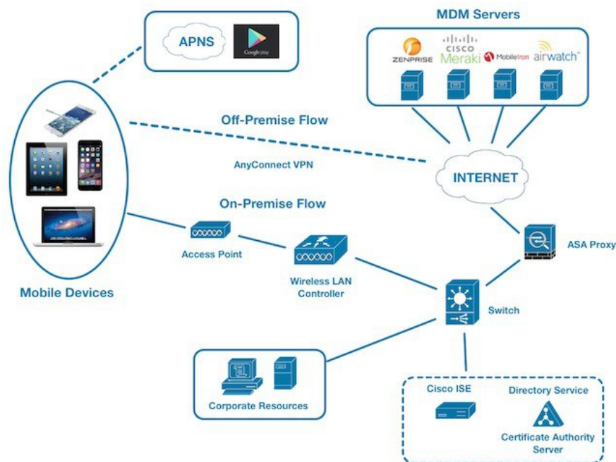
図 44: MDM の Cisco ISE との相互運用性
