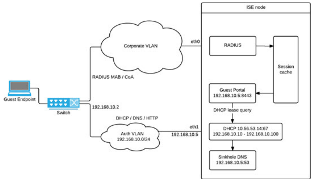
図 1: Cisco ISE ノードに接続された認証 VLAN
