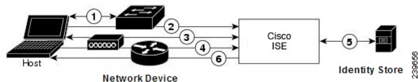
図 2: EAP を使用する RADIUS ベースの認証
