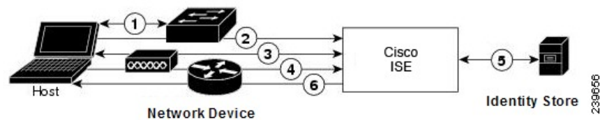
図 2: EAP を使用する RADIUS ベースの認証
