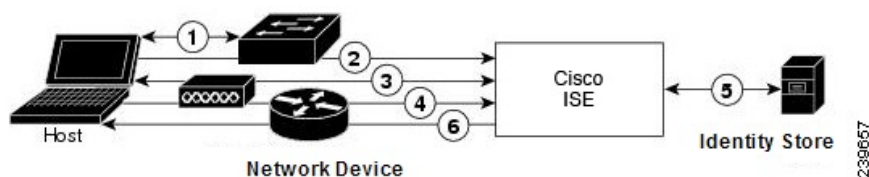
図 1: EAP を使用しない RADIUS ベースの 認証
