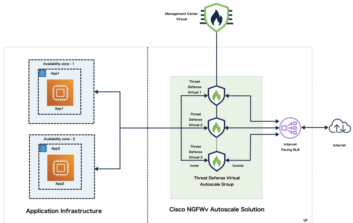
図 1: NLB を使用した Threat Defense Virtual Auto Scale ソリューション
