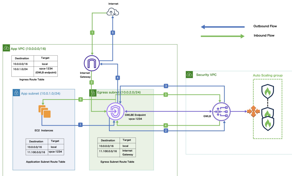
図 3: GWLB を使用した Threat Defense Virtual Auto Scale ソリューション
