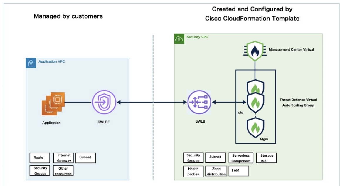
図 2: GWLB を使用した Threat Defense Virtual Auto Scale ソリューション
