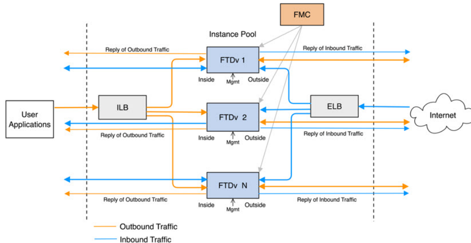
図 4 : Secure Firewall Threat Defense Virtual Auto Scale の導入例の図
