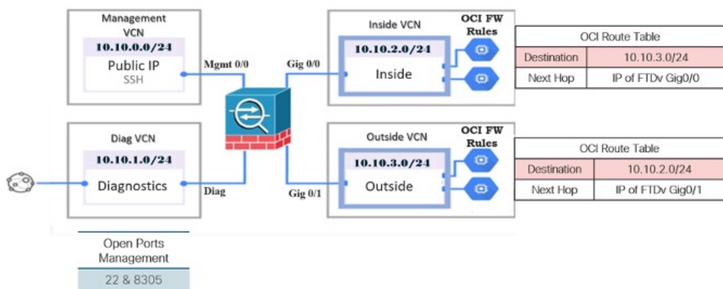
図 1: 4 つの VCN のサブネットを使用した OCI への Threat Defense Virtual の展開の例
