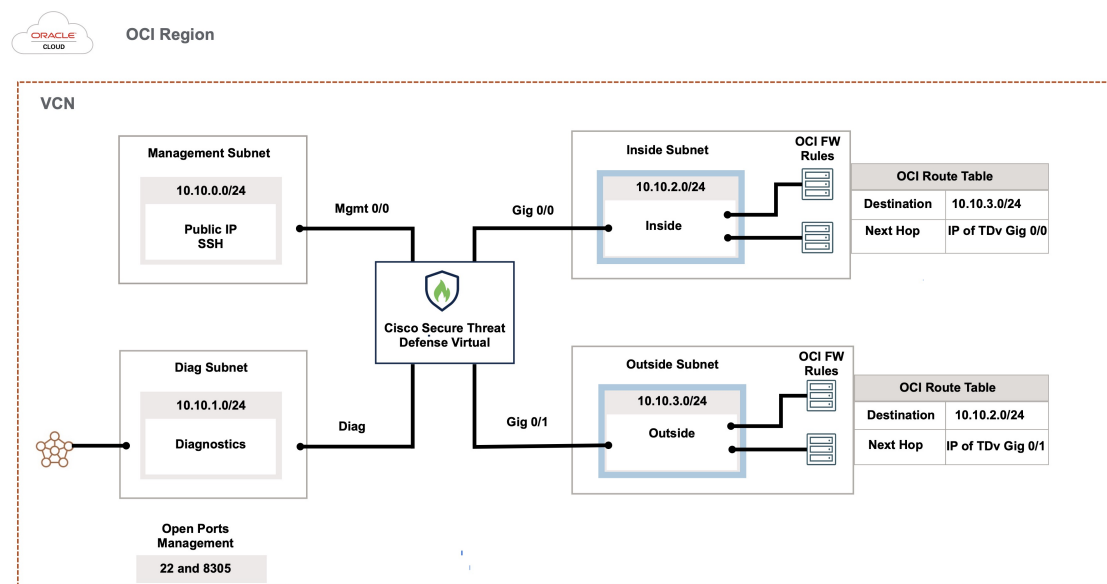
図 2: VCN の 4 つのサブネットを使用した OCI への Threat Defense Virtual の展開の例
