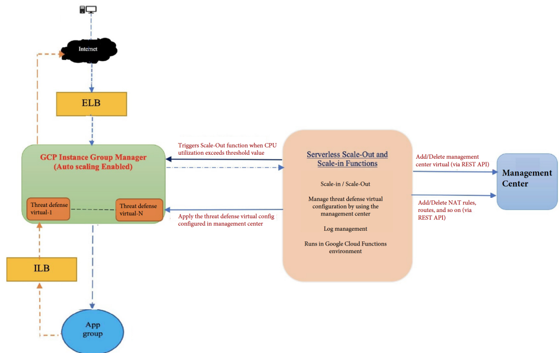
図 5: Auto Scale ソリューションの概要
