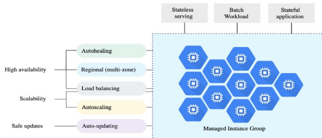
図 4: インスタンスグループの機能
