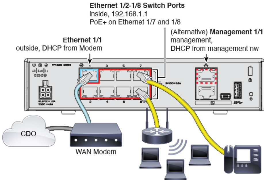
図 5: Firepower 1010 のケーブル配線
