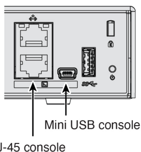
図 7: コンソールポート
