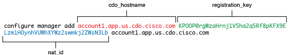
図 27 : configure manager add コマンドコンポーネント
