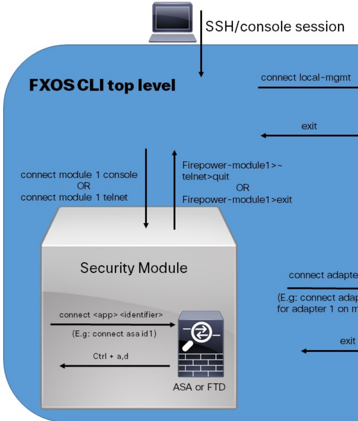
図 1 : Firepower 4100/9300 FXOS CLI 接続図
