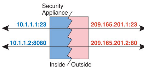
図 15: ポート変換を設定したスタティック NAT の一般的なシナリオ
