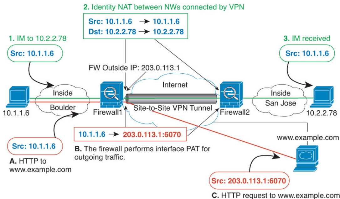
図 25: サイトツーサイト VPN のためのインターフェイス PAT およびアイデンティティ NAT
