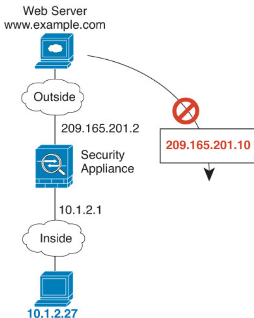
図 12: マッピングアドレスへの接続開始を試みているリモート ホスト
