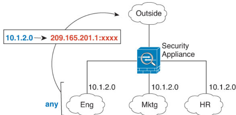
図 10: 任意のインターフェイスの指定
