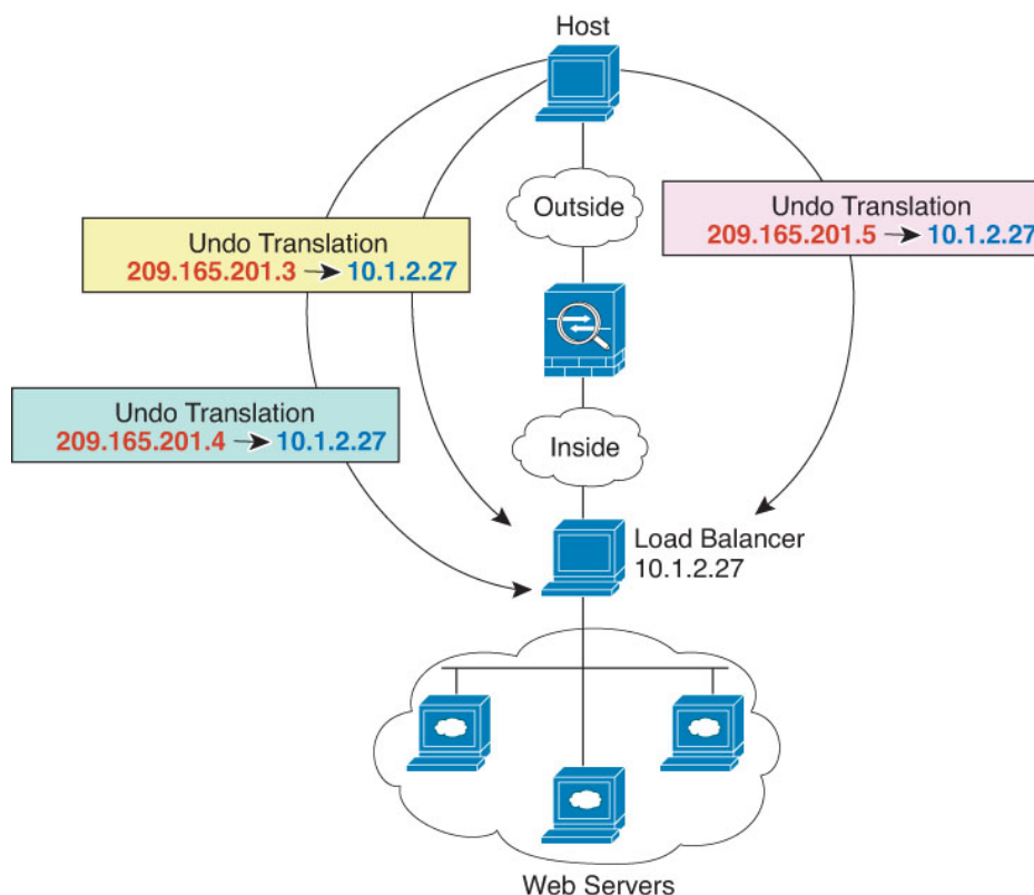
図 17:1 対多のスタティック NAT の例
