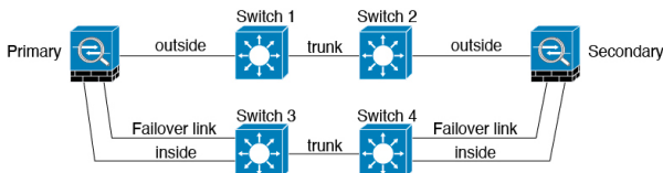
図 6: セキュア スイッチを使用した接続
