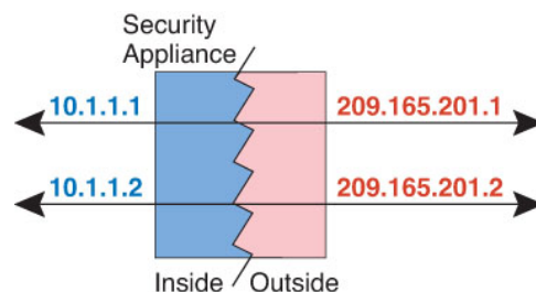
図 14:スタティック NAT
