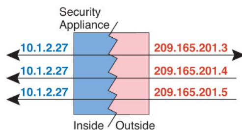
図 16: 1 対多のスタティック NAT
