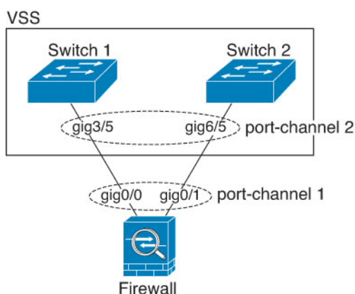
図 7: VSS/vPC への接続
