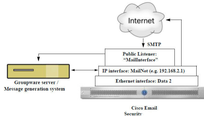
Figure 3: 2つだけイーサネットインターフェイスを持つ電子メールゲートウェイモデル上のパブリックリスナー
