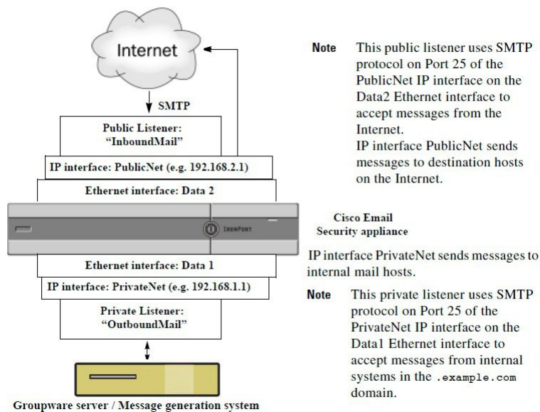
図3: 2つだけイーサネットインターフェイスを持つアプライアンスモデル上のパブリックリスナー
