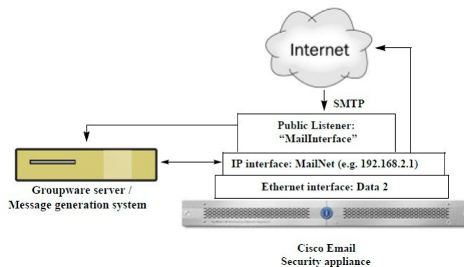
図3: 2つだけイーサネットインターフェイスを持つアプライアンスモデル上のパブリックリスナー
