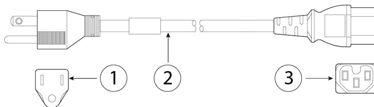
図 28: 北米 CAB-9K12A-NA
