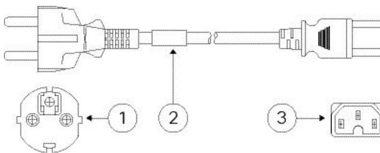
図 27: 韓国 CAB-9K10S-KOR
