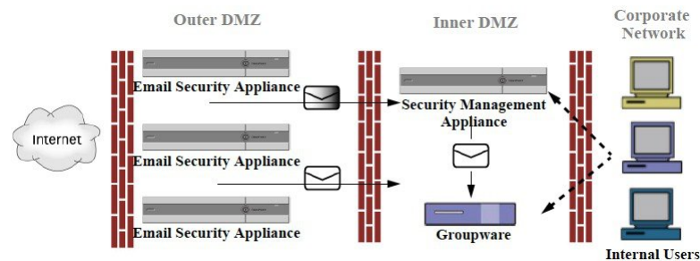
Figure 1: Cisco Secure Email and Web Manager による一般的なネットワーク設定
