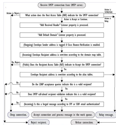
Figure 6: 電子メールパイプライン：電子メール接続の受信
