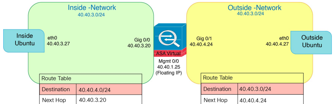
図 2: OpenStack への ASA 仮想 の導入例
