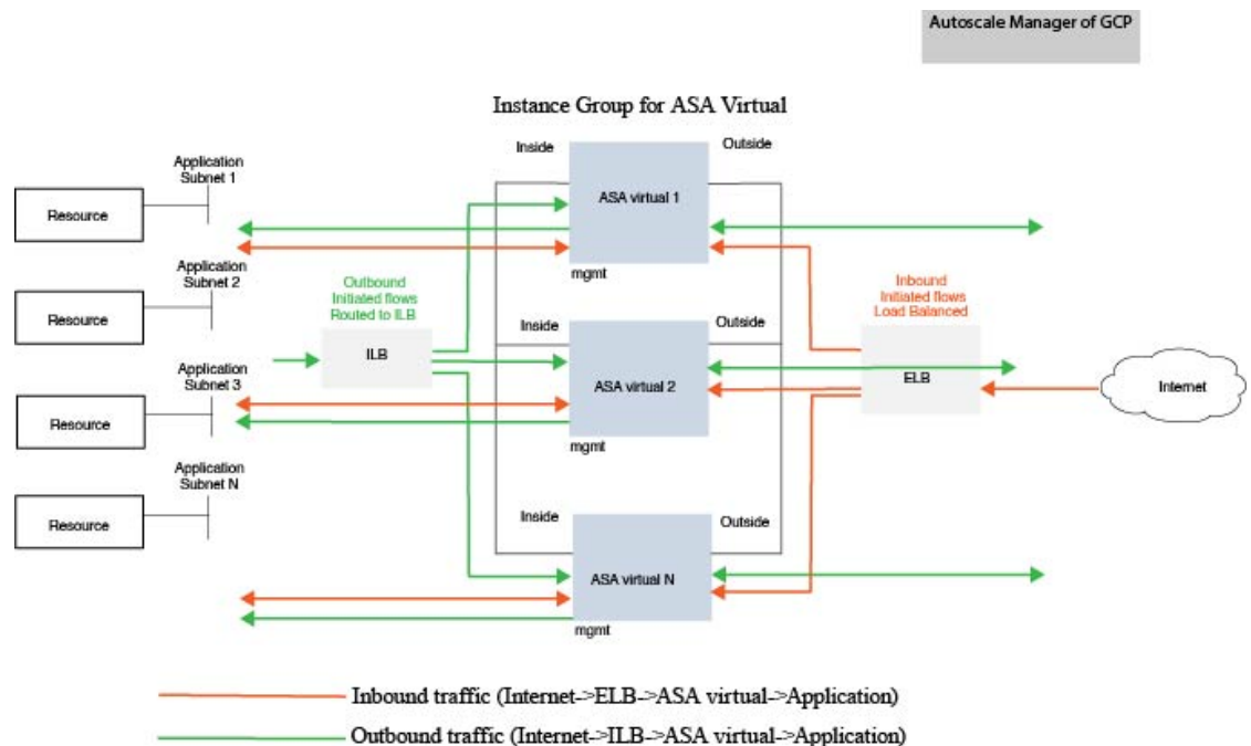
図 1: ASA 仮想 自動スケールのユースケース
