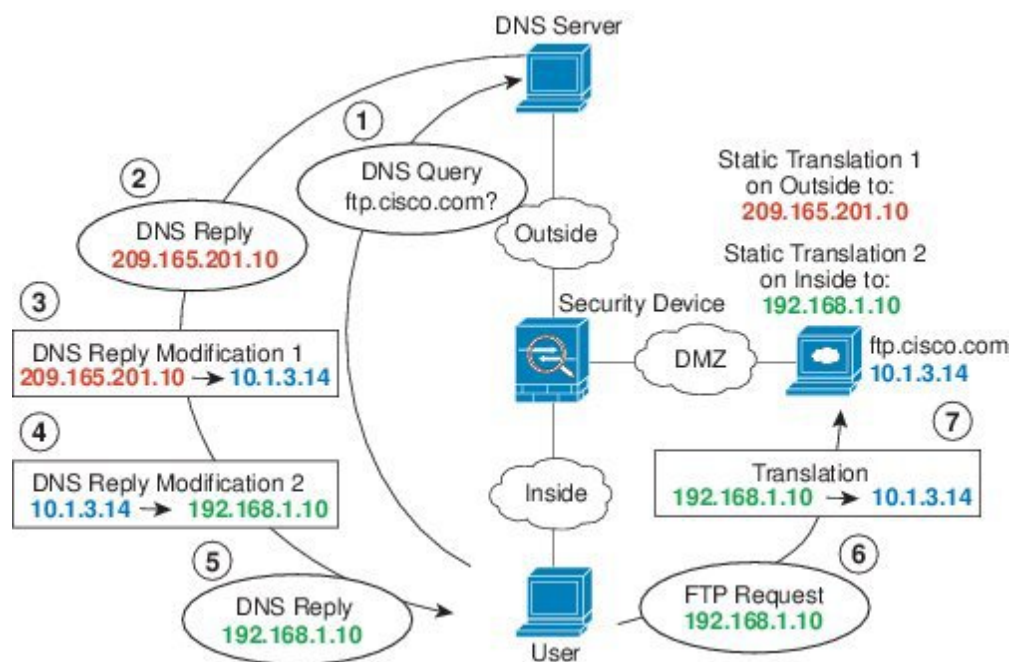
図 18: DNS 応答修正：別々のネットワーク上の DNS サーバ、ホスト、およびサーバ
